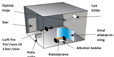
Brandtest for røgd udvikling Kabler med minimal røgd udvikling. Standard IEC 61034-2 og EN 50268-2
